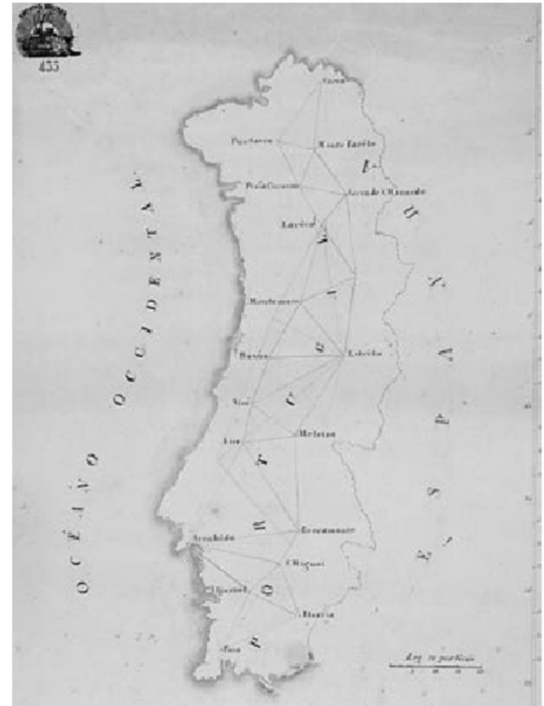
Fig.1. Primeiro esquema de triangulação projectado por Ciera após as expedições geográficas de 1790-91. Reprodução do original pertencente à Direcção dos Serviços de Engenharia.
