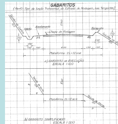
Exemplo de projecto de perfil transversal
