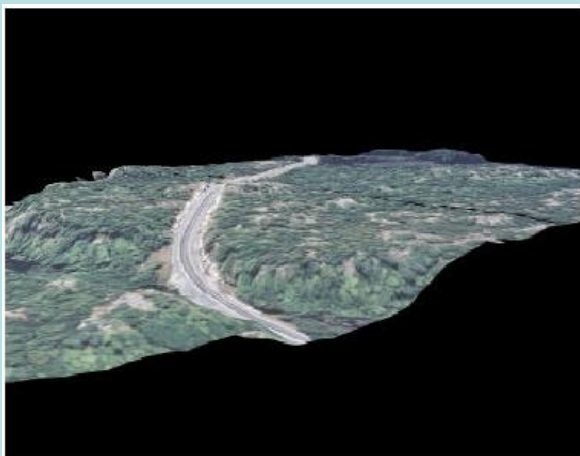
Boa coordenação do traçado em planta e perfil longitudinal
