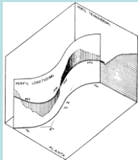
eixo do traçado
