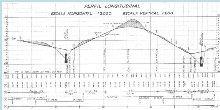
Exemplo de projecto de rasante (perfil longitudinal)
