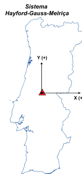
Fig. 8 - Sistemas de coordenadas utilizando o Datum 73, com a representação da origem e orientação dos eixos do referencial e ponto de fixação do elipsoide de referência (triângulo vermelho).
