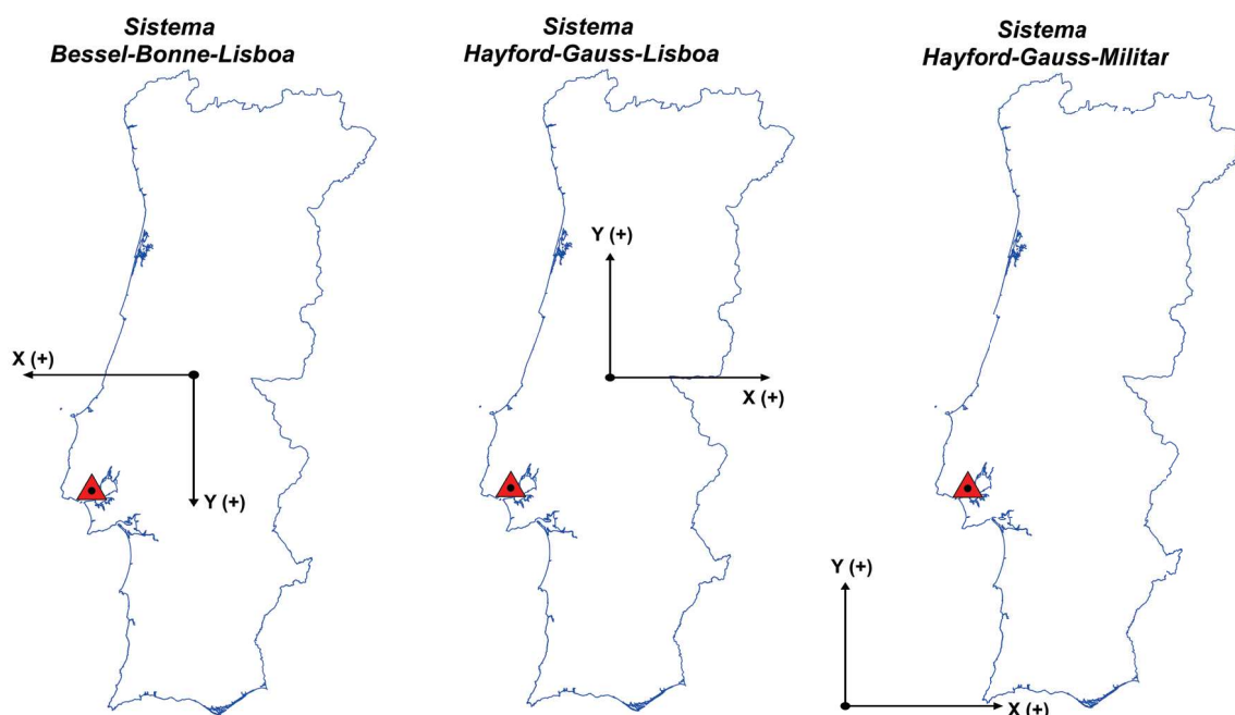
Fig. 7 - Sistemas de coordenadas utilizando o Datum Lisboa, com a representação da origem e orientação dos eixos do referencial e ponto de fixação do elipsoide de referência (triângulo vermelho).
