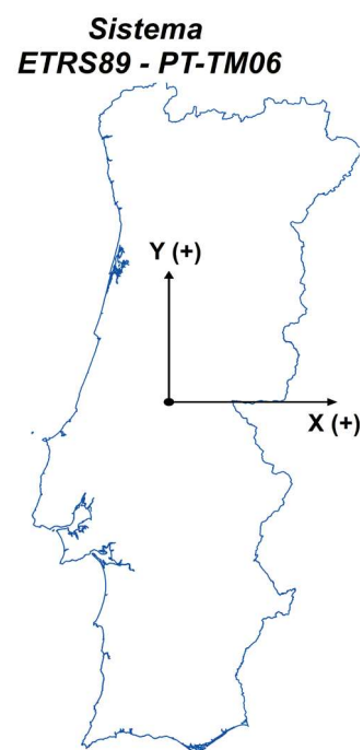
Fig. 10 - Sistemas de coordenadas utilizando o sistema ETRS89-TM06 com a representação da origem e eixos do referencial.
